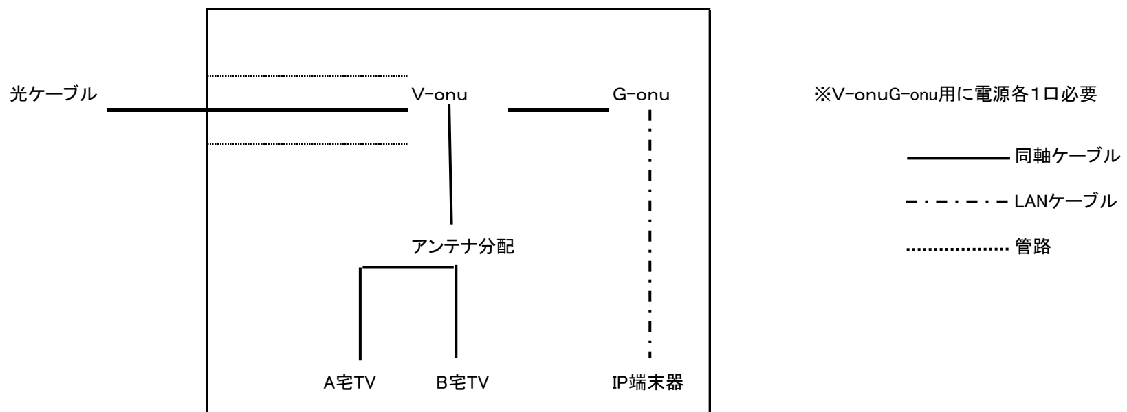
図(テレビアンテナを共有スペースに設置する場合)
